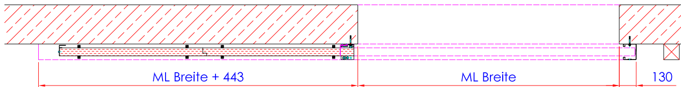
Schnitt B-B
