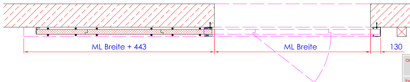
Schnitt B-B
