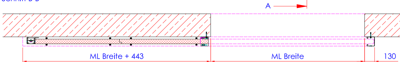
Schnitt B-B
