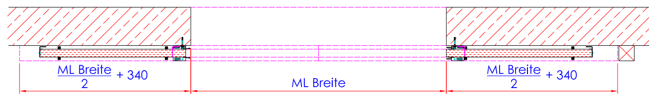
Schnitt B-B
