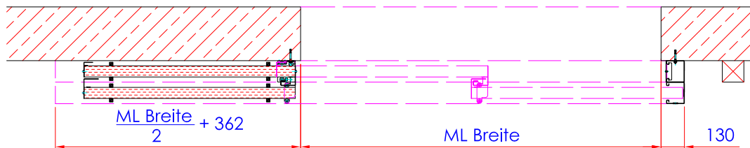
Schnitt B-B
