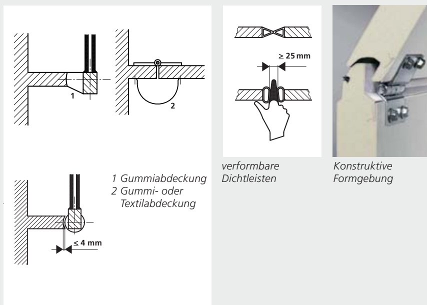
verformbare Abdeckung
